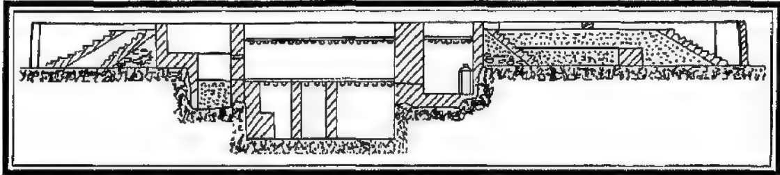
(شكل ٤٥) مسقط رأسى للتصميم التالى للمقبرة ٢٠٢٨ فى سقارة.
